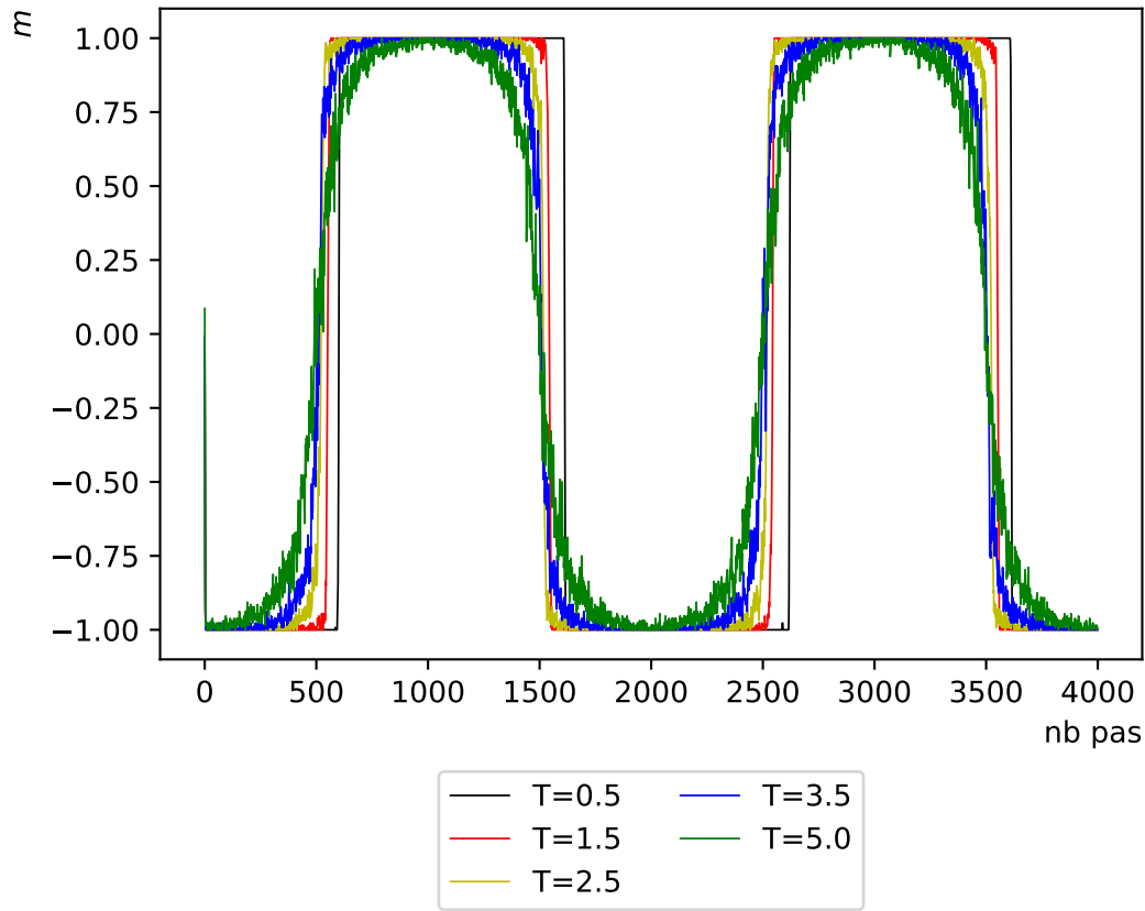
Aimantation d'un réseau de taille L=16 dans un champ magnétique d'amplitude h=10
